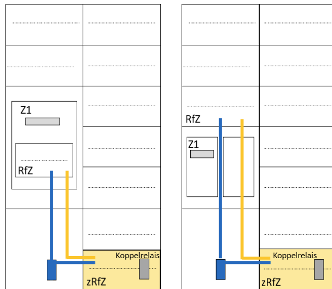
Abbildung 9: Bestandszählerplatz mit einem 1-feldrigen Zählerfeld
