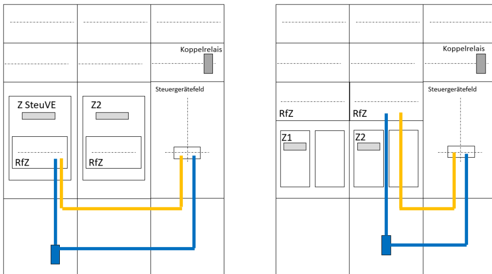
Abbildung 10: Bestandszählerplatz mit einem Steuergerätefeld
