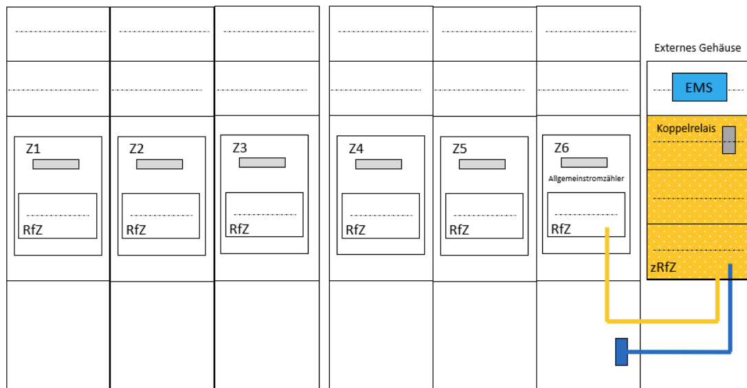
Abbildung 11: Bestandszählerplätze ohne zusätzlichen Zählerplatz bzw. Steuergerätefeld
