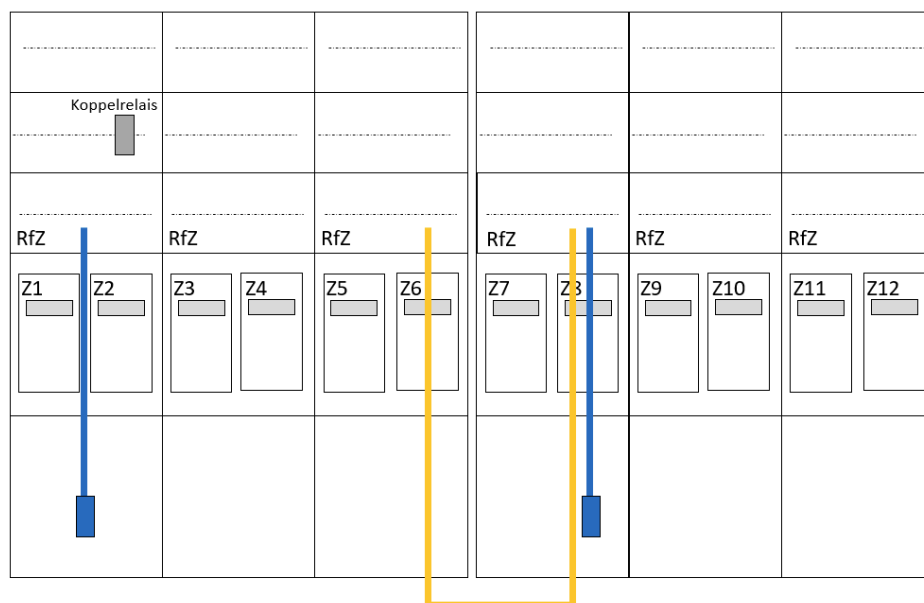
Abbildung 12: Bestandszählerplätze ohne zusätzlichen Zählerplatz bzw. Steuergerätefeld
