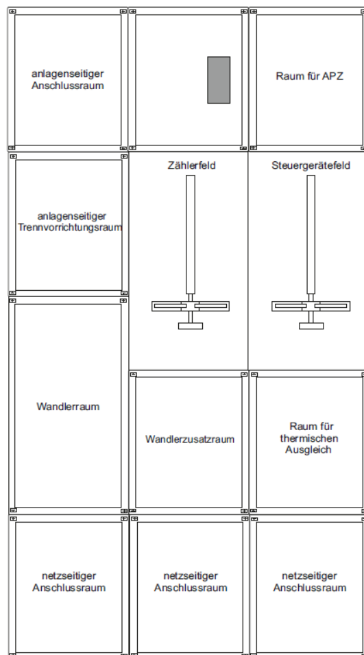
Abbildung 8: Bsp. Wandlermessung 200 A in Neuanlagen
